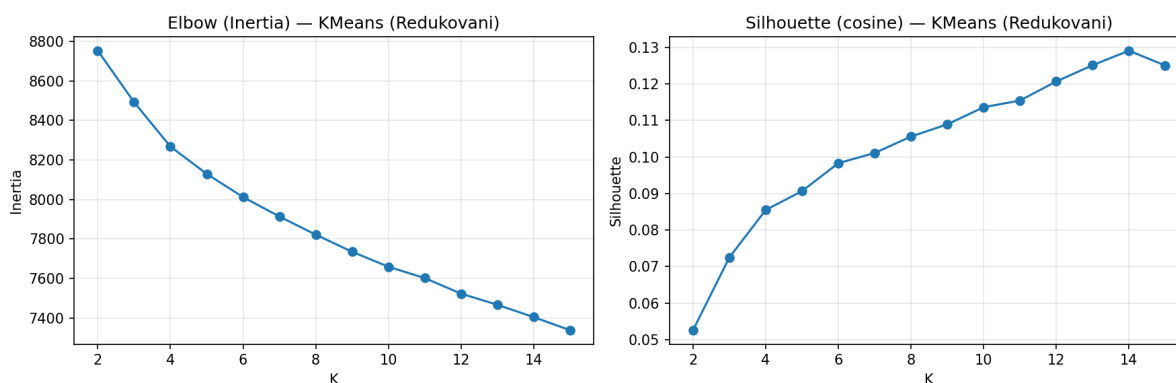
Slika 20: Elbow i Silhouette analiza za određivanje optimalnog K – redukovani atributi (SVD)
